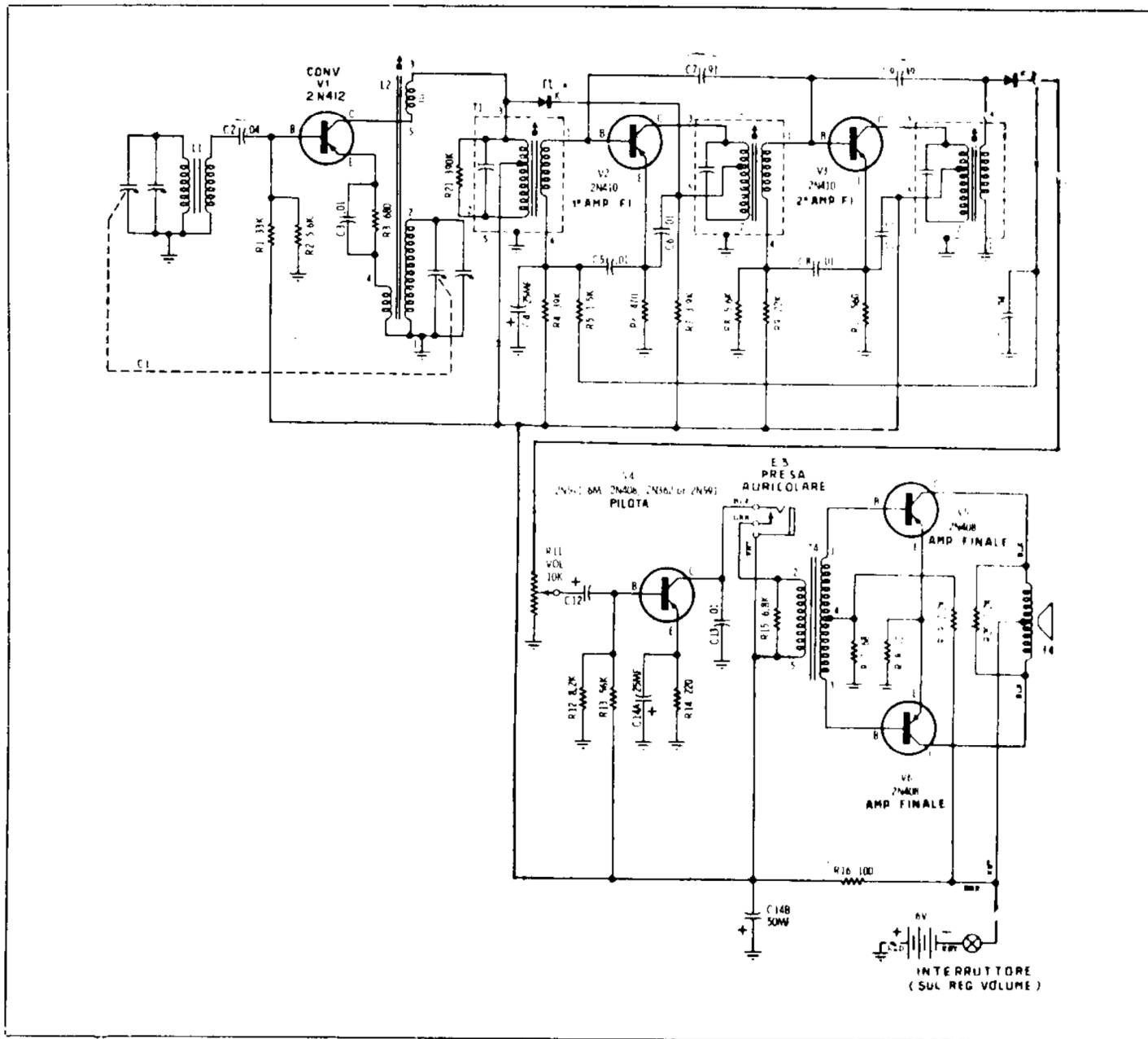
Fig. 8-6. - Radioricevitore portatile a sei transistori (Motorola 6X28). Questo ricevitore ha uno stadio di uscita in controfase impiegante un altoparlante con bobina da 300 \Omega e con presa centrale. Si elimina in tal modo la necessit  del trasformatore di uscita.
